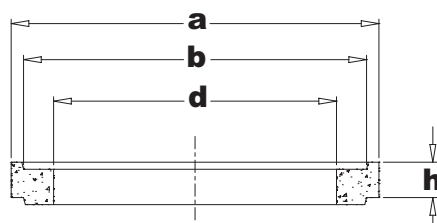
type AR-V 800 - 60/100
